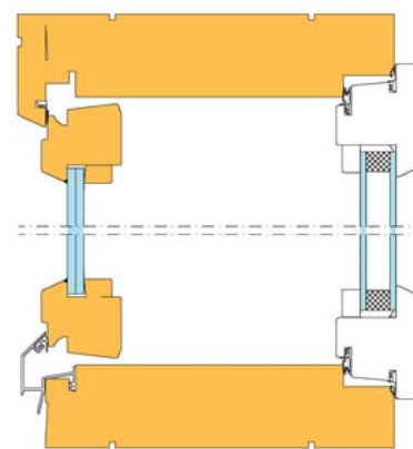
MSE 210. Однокамерный стеклопакет со стёклами 6 мм и 4 мм и дистанционной рамкой 12 мм. В уличной створке ламинированное стекло 3 мм + 3 мм с плёнкой 0,38 мм.
