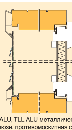
Разрез клапанной створки «ДОМУС ALU»
