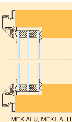
Разрез глухого оконного блока «ДОМУС ALU»
