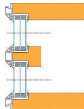
Глухой деревоалюминиевый оконный блок Домус МЕК с промежуточным импостом коробки
