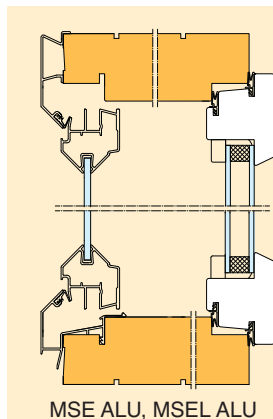
Разрез оконного блока «ДОМУС ALU»
